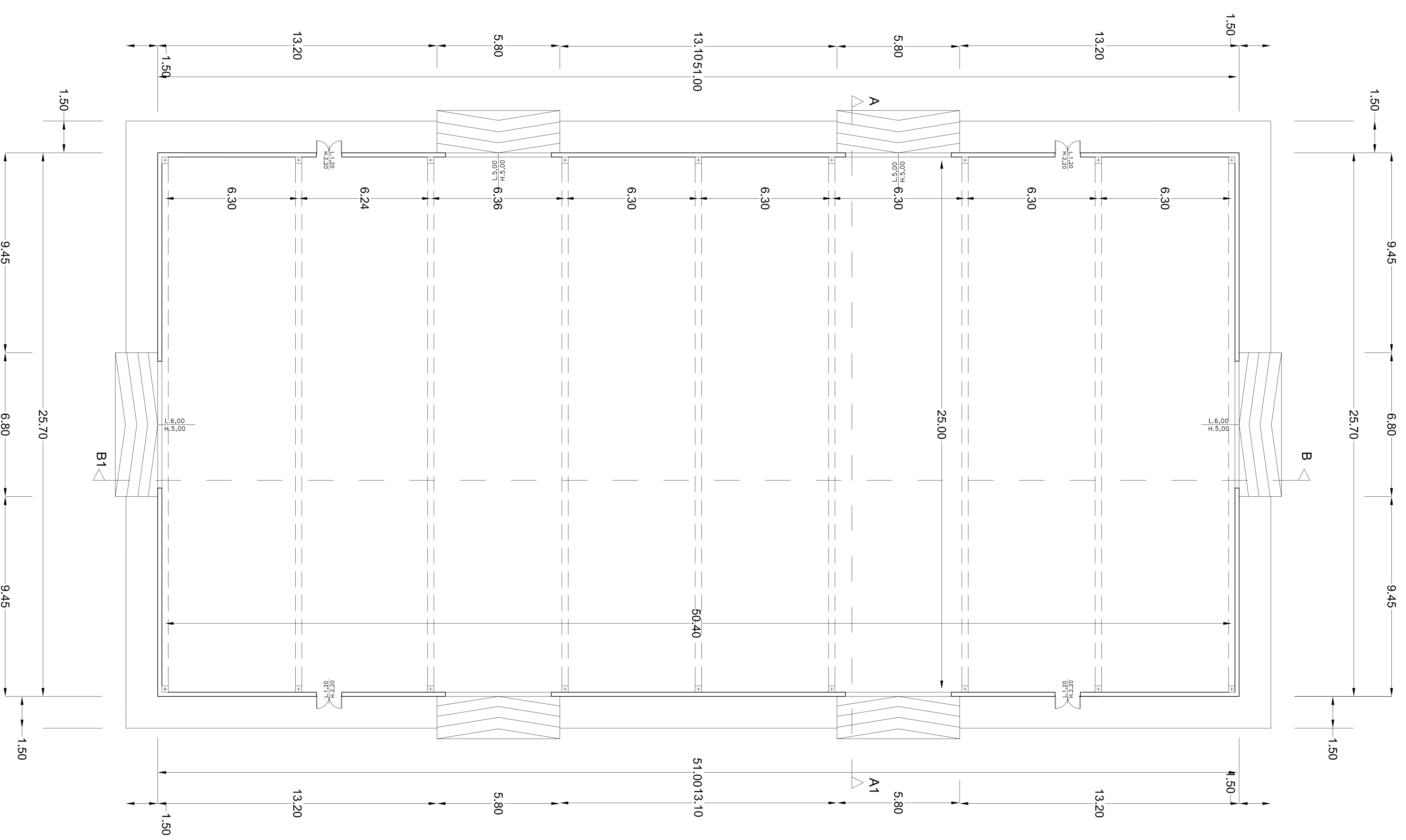
PIANTA PIANO TERRA
